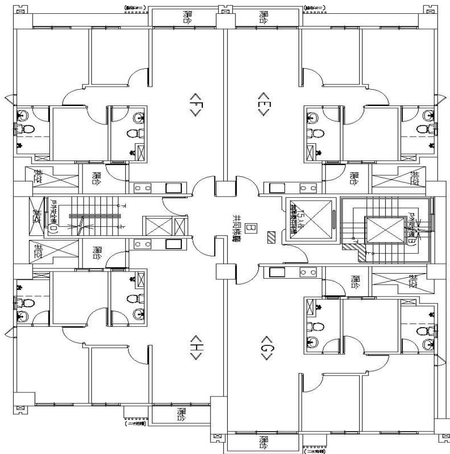
肆到陸層平面圖-施工
