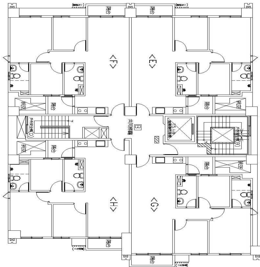
屋突一層、柒層平面圖-施工
